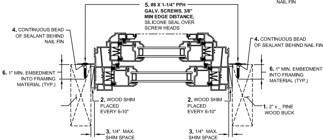
SIDE JAMB
